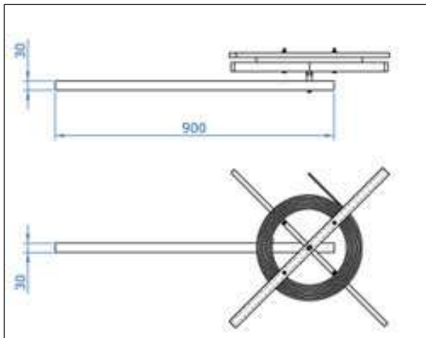
URZĄDZENIE DO ODWIJANIA TAŚMY PRZEWODZĄCEJ
