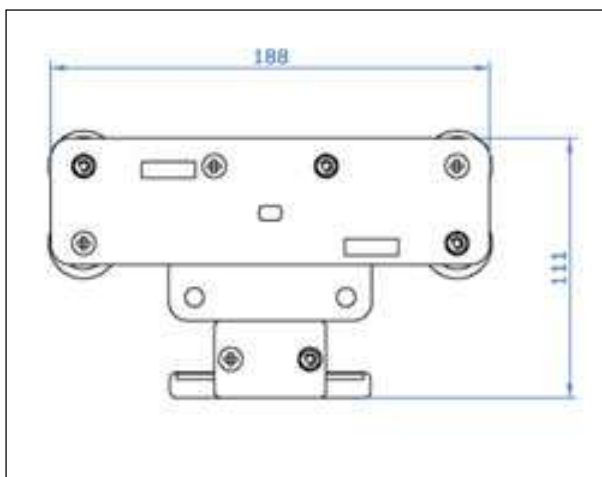
WÓZEK DO WCIĄGANIA TAŚMY PRZEWODZĄCEJ
